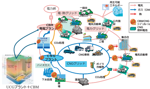
CNG (圧縮天然ガス) による二つのエネルギー供給モデル
