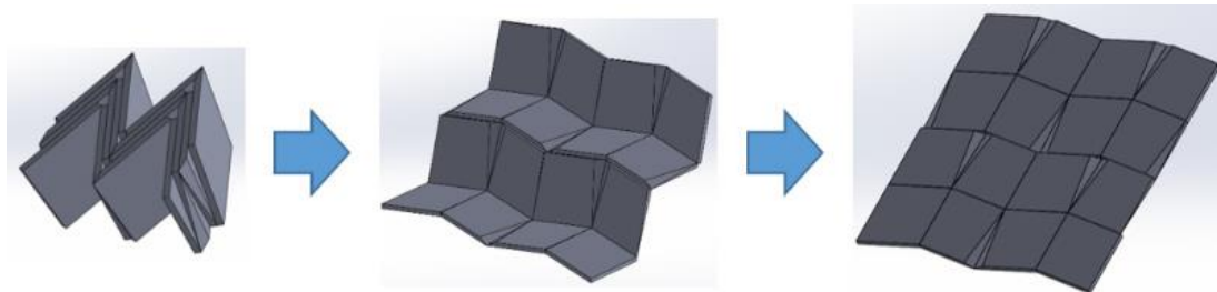
二次元展開板構造の展開の様子
